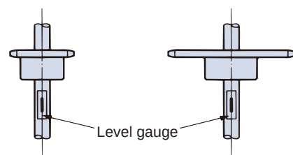
Fig. 15 Horizontal precision
